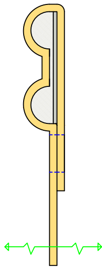
Snap-ring inox double bourrelet sous tresse de verre
